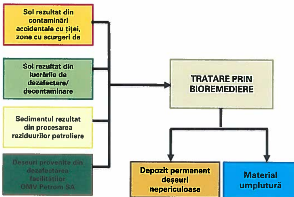
Diagrama fluxurilor procesului tehnologic
