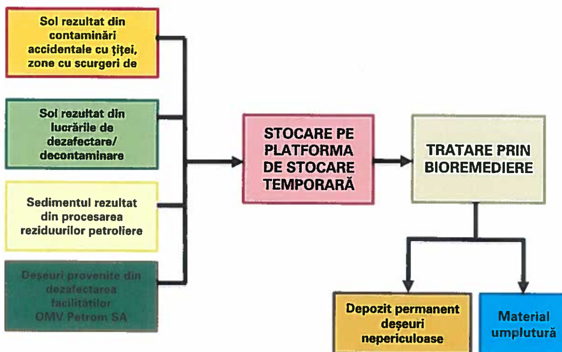
Diagrama fluxurilor procesului tehnologic
