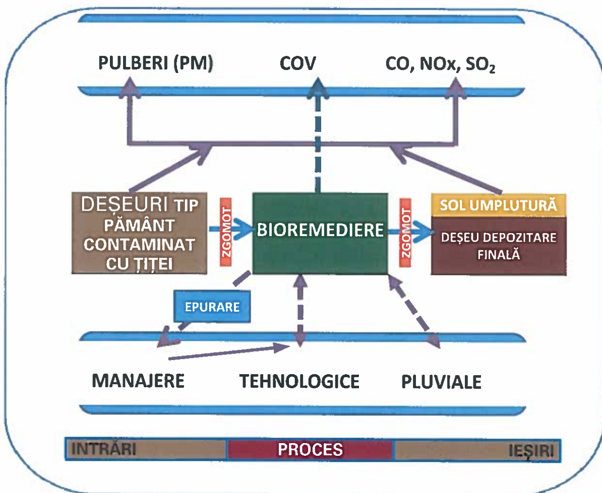
Figura 4. – Diagrama emisiilor de proces tehnologic
