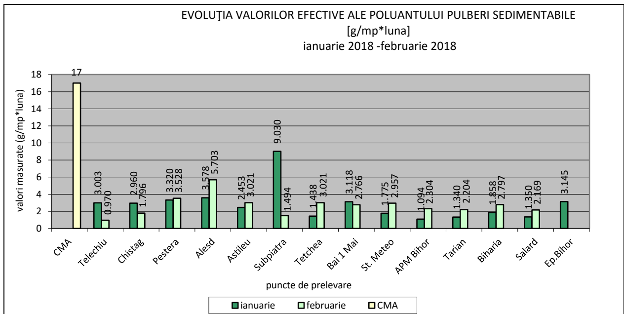
Fig.1.Pulberi sedimentabile
