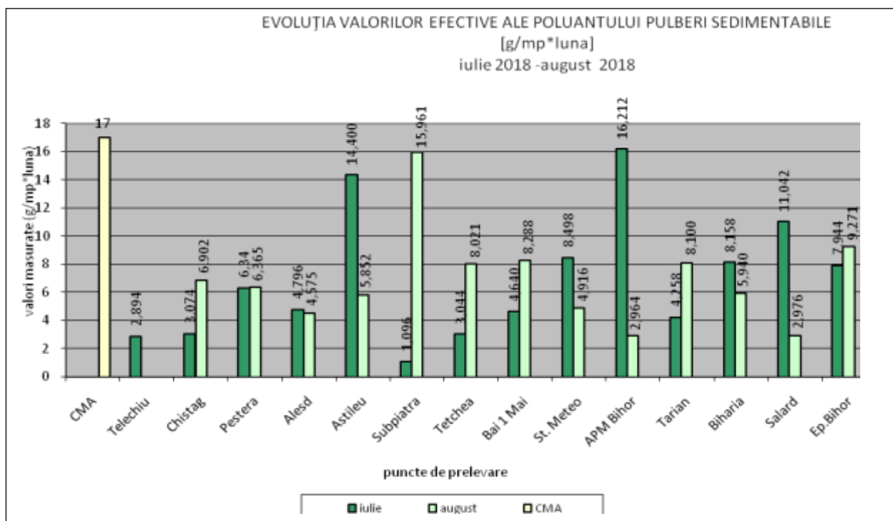
Fig.2.1.1.1. Pulberi sedimentabile
