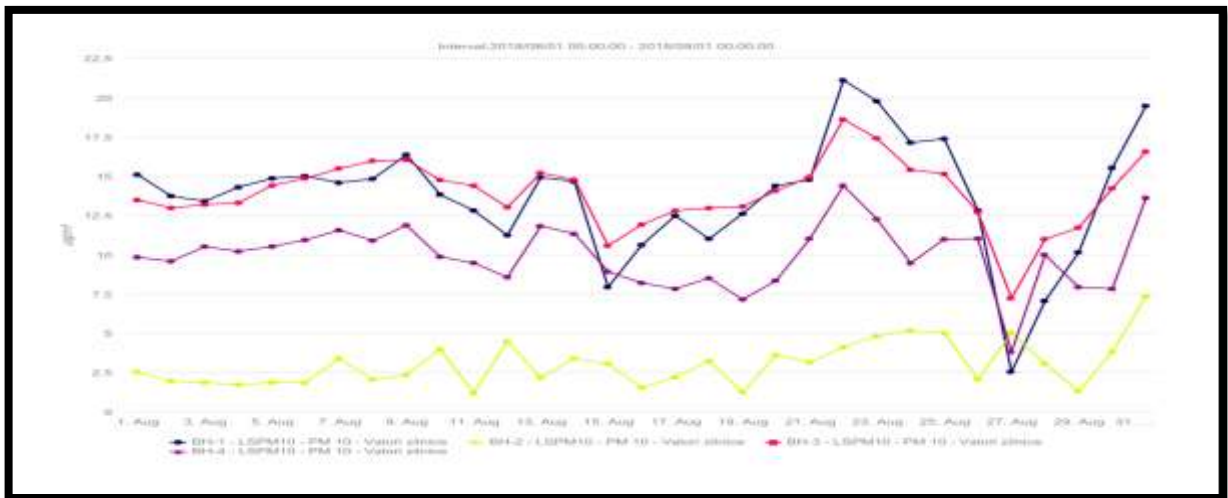
Fig.2.2.6. Concentrații PM 10
