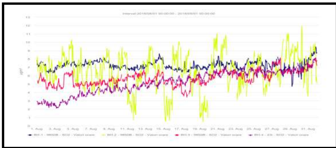
Fig.2.2.3. Concentrații SO_2
