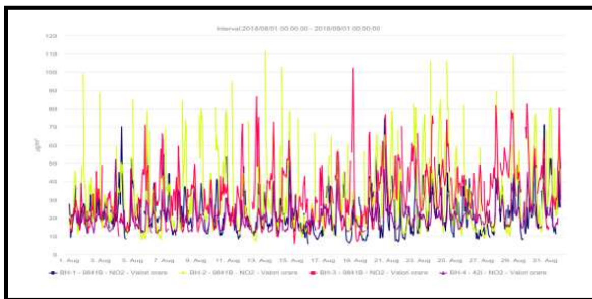
Fig.2.2.4. Concentrații NO_2
