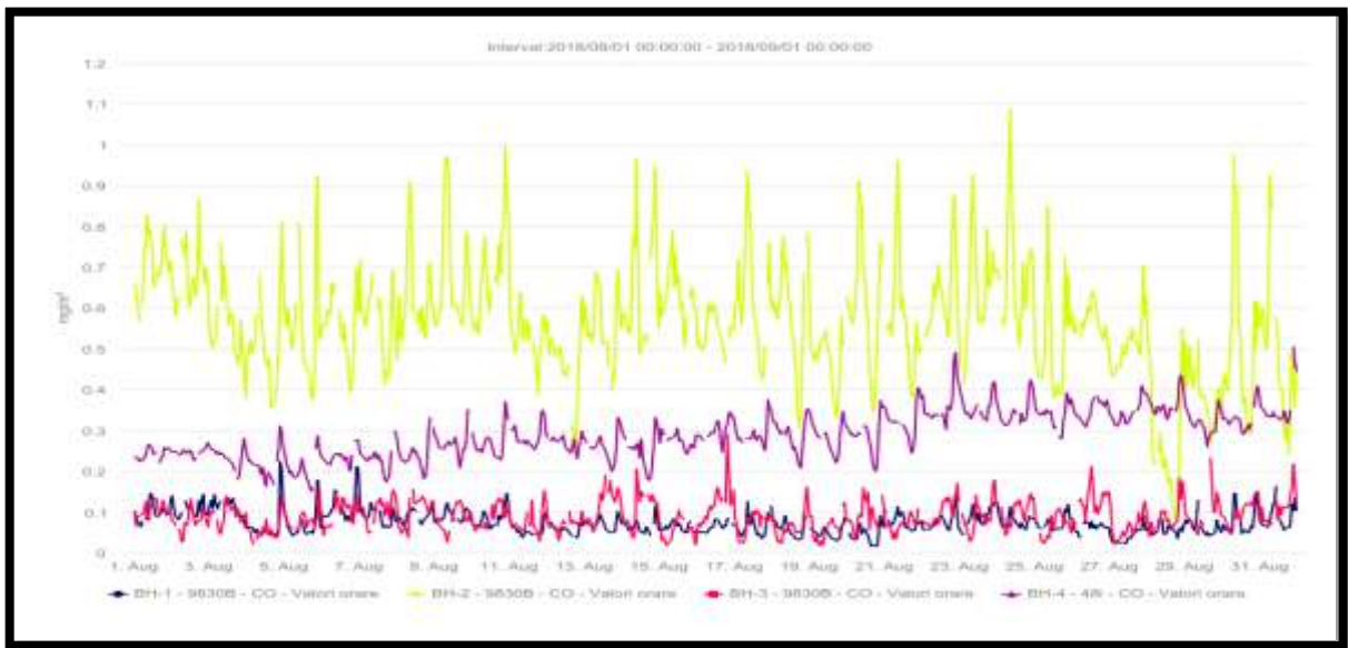
Fig.2.2.5. Concentrații CO
