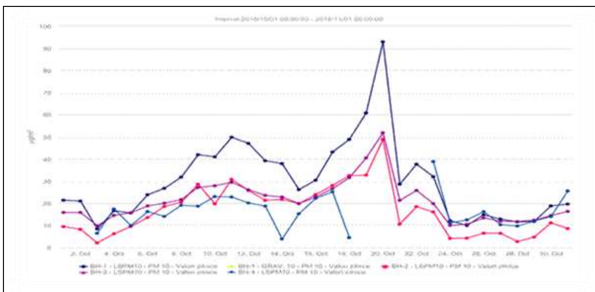
Fig.2.2.6. Concentrații PM 10
