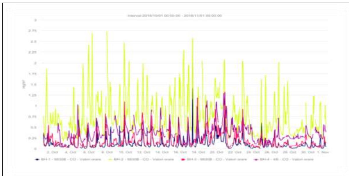
Fig.2.2.5. Concentrații CO
