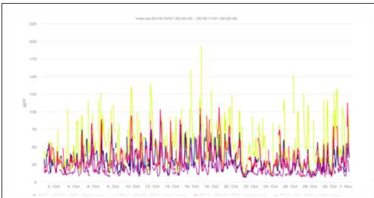
Fig.2.2.4. Concentrații \text{NO}_2
