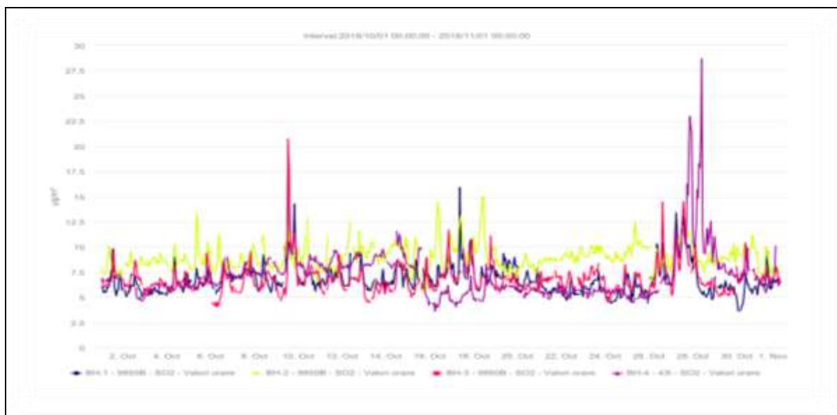
Fig.2.2.3. Concentrații \text{SO}_2
