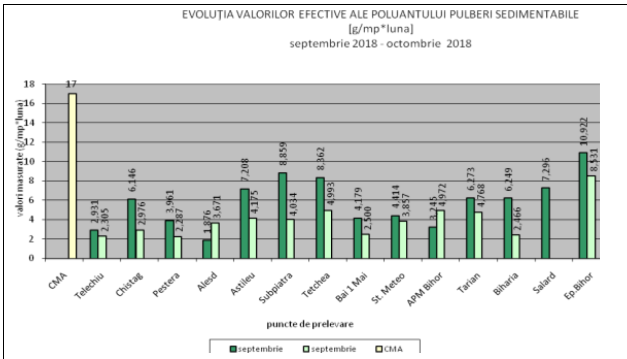
Fig.2.1.1.1.Pulberi sedimentabile
