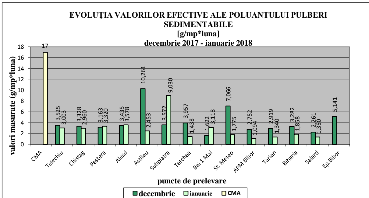
Fig.2. Pulberi sedimentabile
