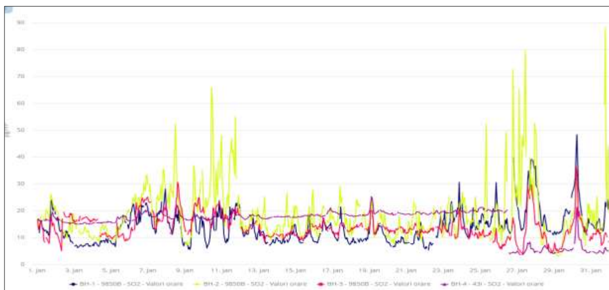
Fig.3. Concentrații SO 2
