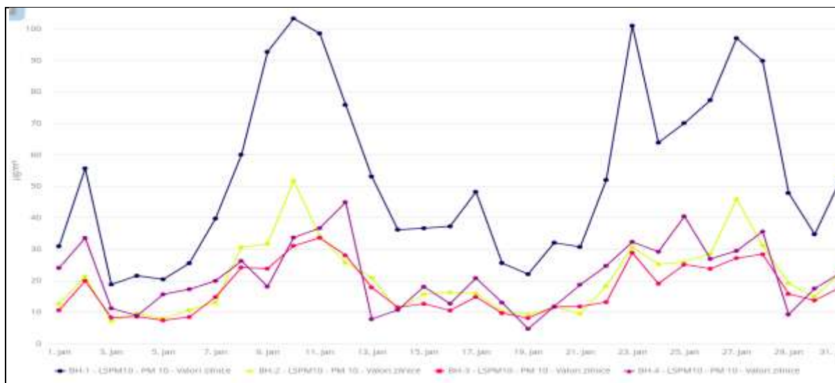
Fig.6. Concentrații PM10
