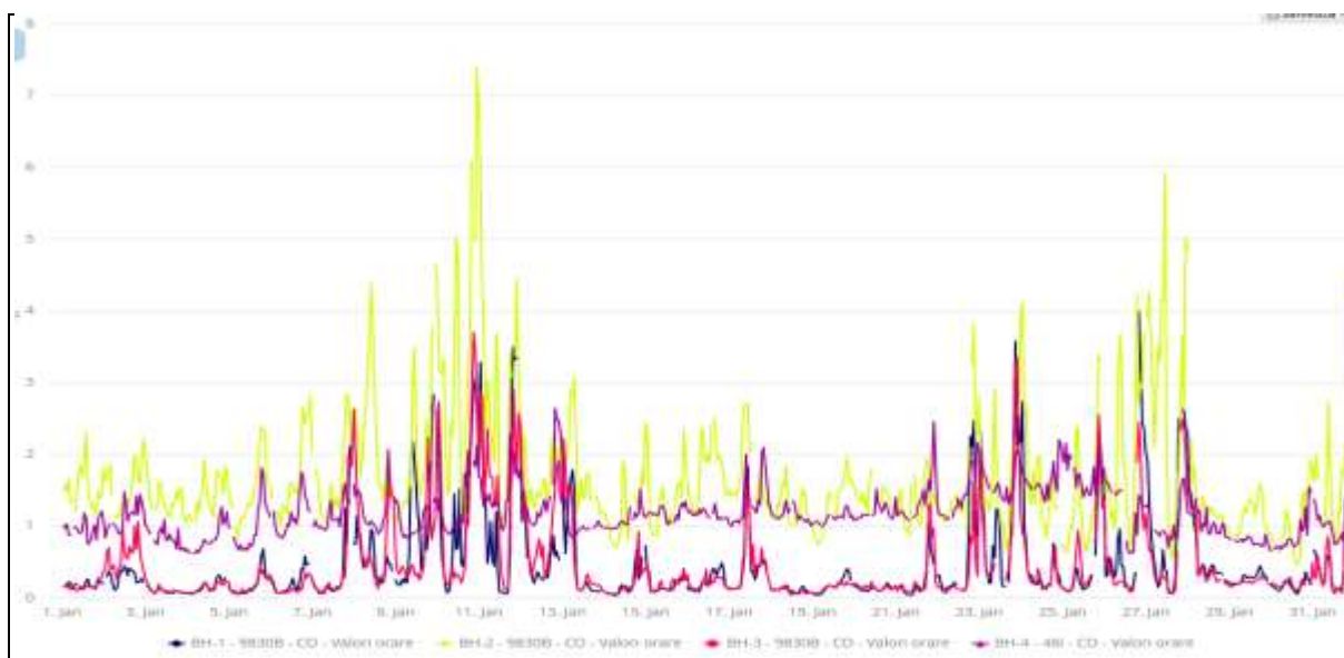
Fig.5. Concentrații CO
