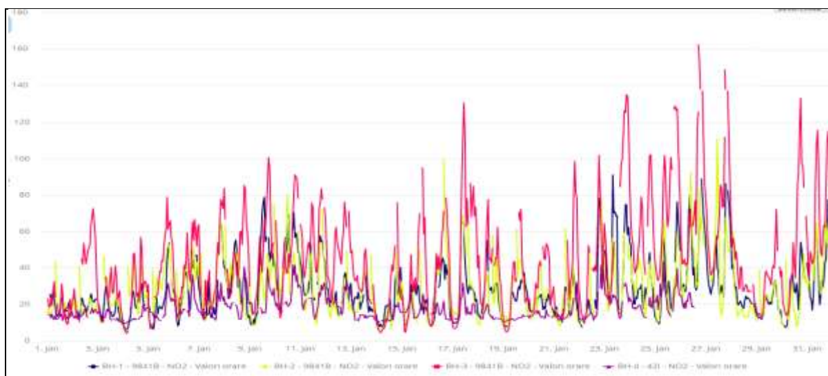
Fig.4. Concentrații NO2
