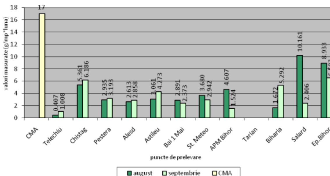
EVOLUȚIA VALORILOR EFECTIVE ALE POLUANTULUI PULBERI SEDIMENTABILE [g/mp*luna] august 2016 - septembrie 2016
