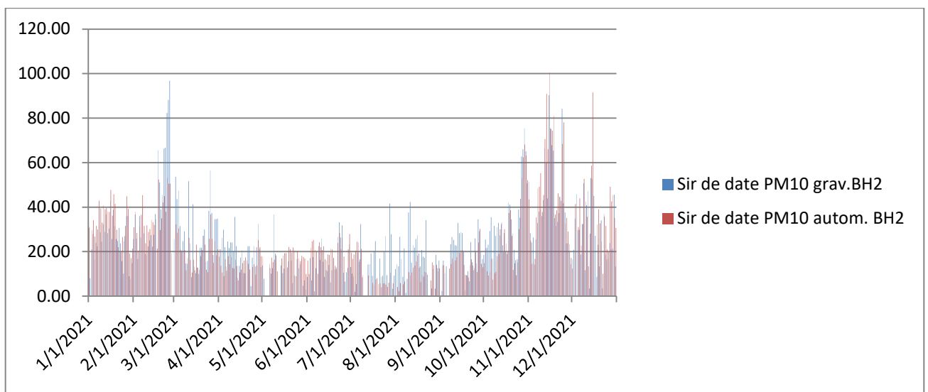
Stația BH 2 , cu determinări de PM 10 (nefelometrice) și gravimetric.
