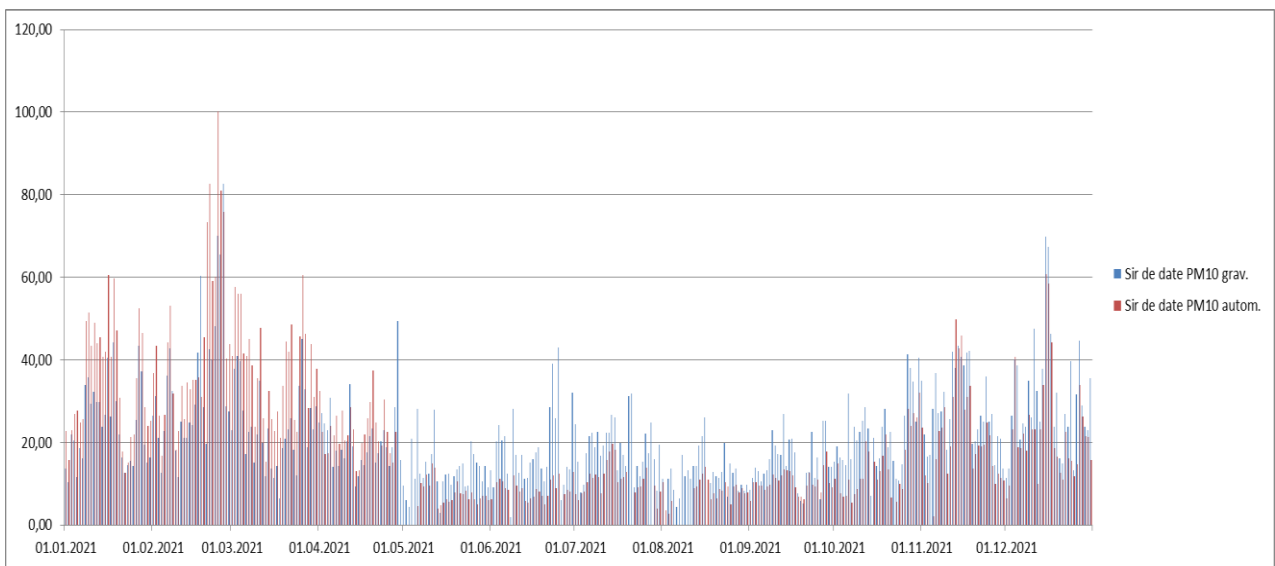
Stația BH 2 , cu determinări de PM 10 (nefelometrice) și gravimetric.
