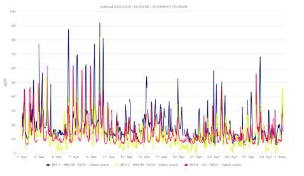
Fig.2.2.7. Concentrații \text{NO}_2
