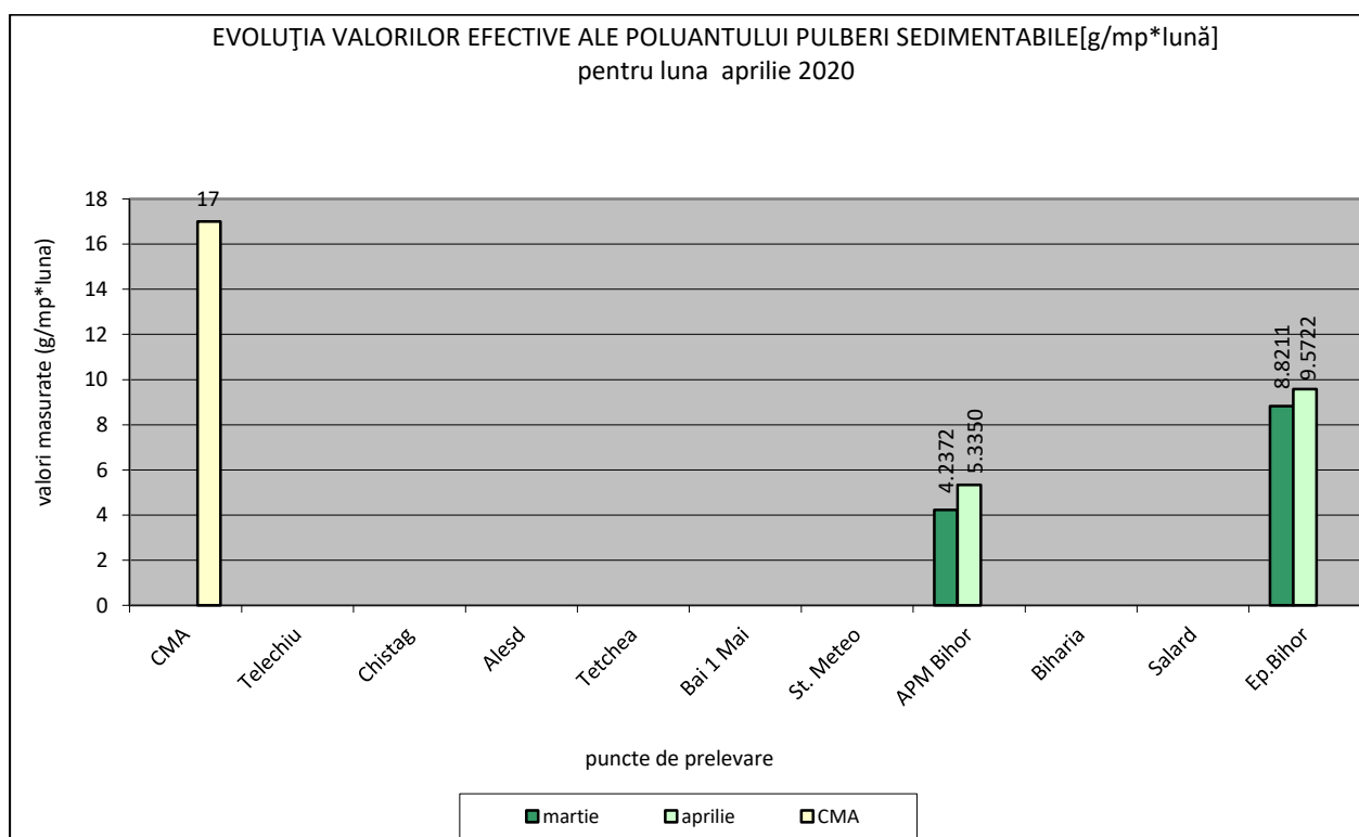
Fig.2.1.1.1.Pulberi sedimentabile
