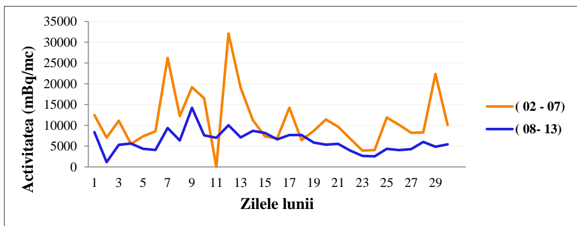
Fig.3.1.2.1. Activitatea specifică beta globală a Radonului
