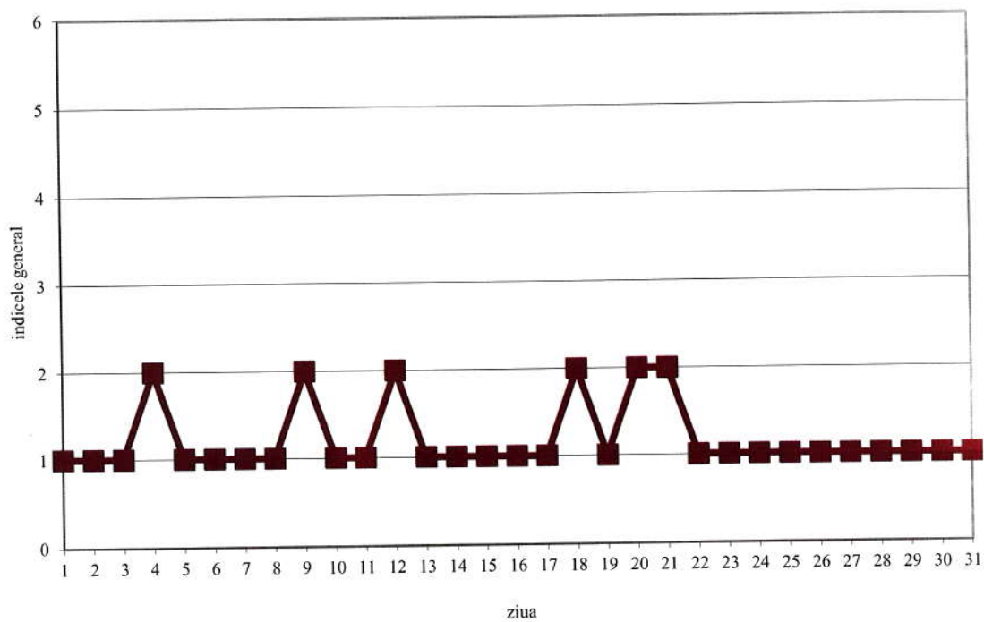
EVOLUȚIA INDICELUI GENERAL LA STAȚIA AUTOMATĂ BH 3 ÎN LUNA decembrie 2022
